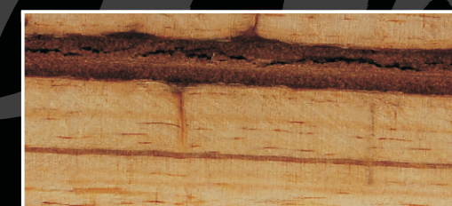
12 Open Pith / Médula abierta
